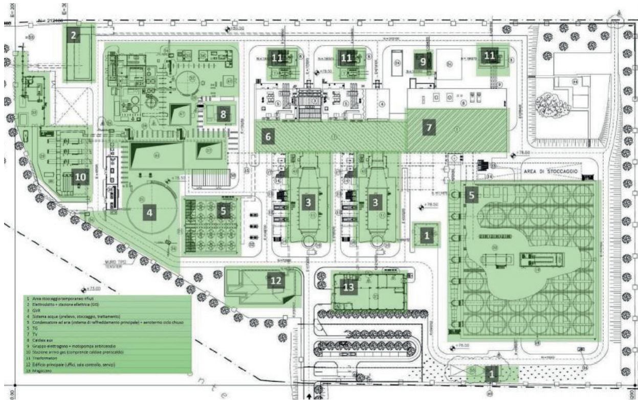
Figura 6 Planimetria della Centrale di Aprilia
