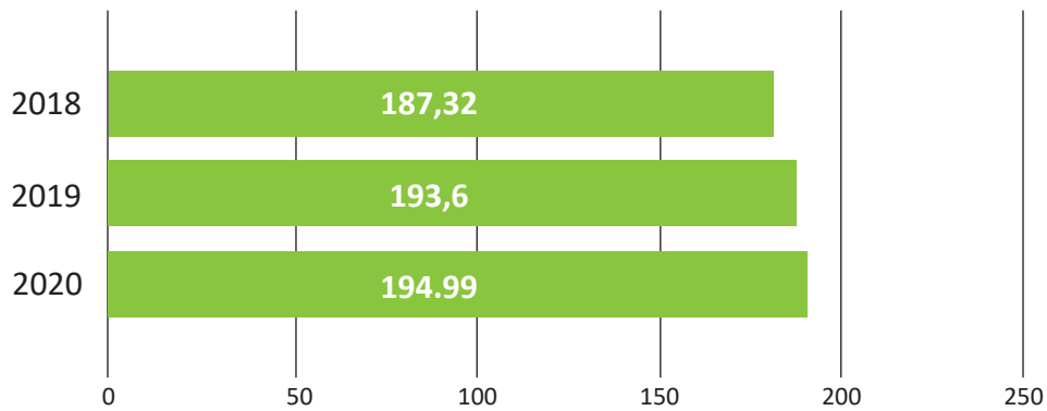
Grafico 6 - Consumo specifico di gas naturale - Sm 3 /MWh
