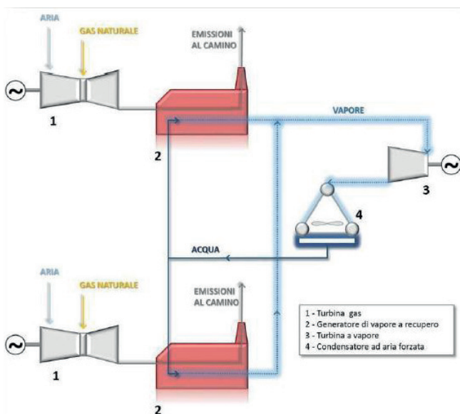
Figura 7 Diagramma del funzionamento di una Centrale a ciclo combinato
