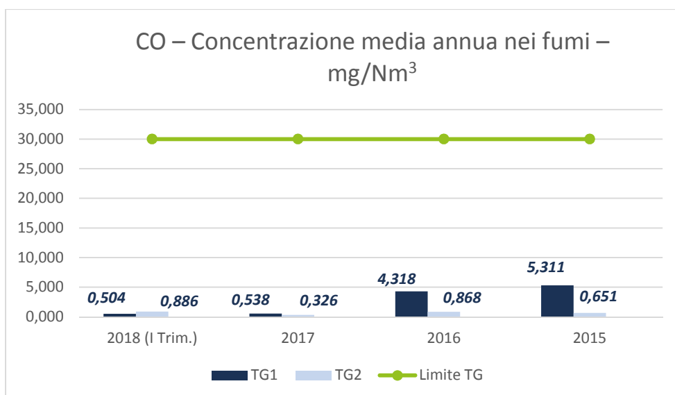
Grafico 4 – Concentrazione CO nei fumi
