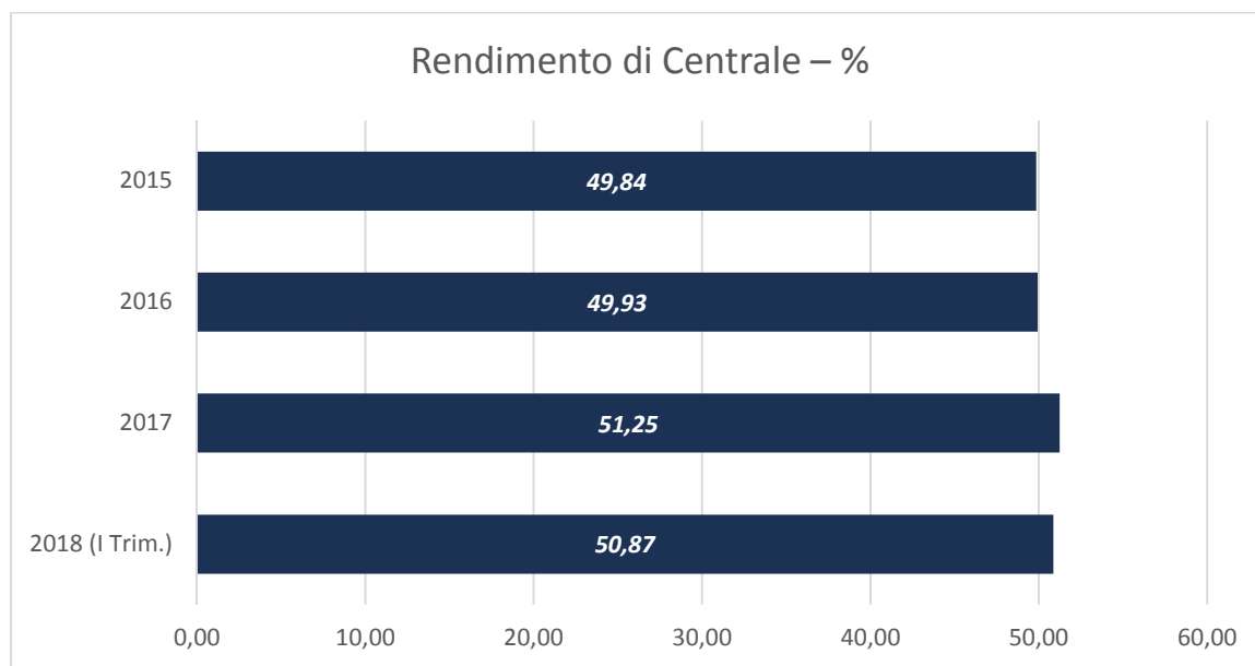
Grafico 7 – Rendimento di centrale
