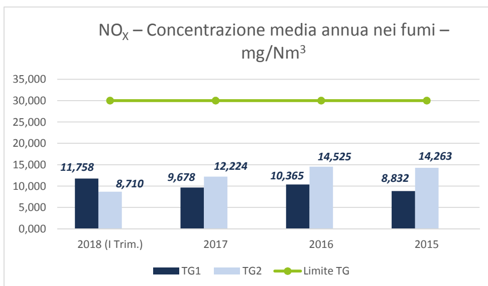
Grafico 3 – Concentrazione NO x nei fumi
