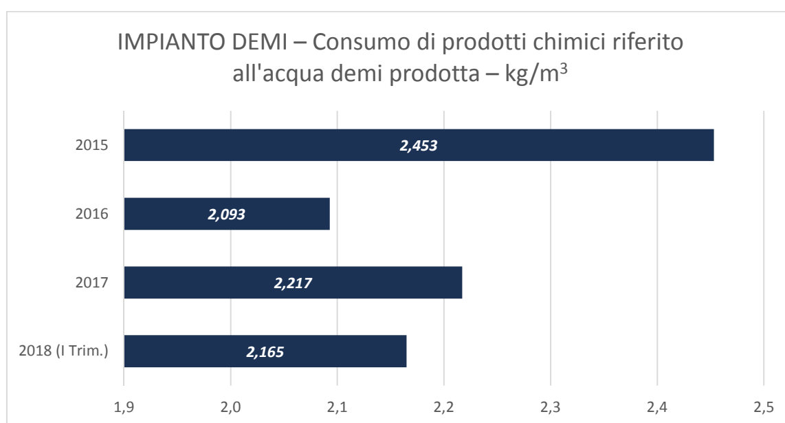
Grafico 14 – Utilizzo di prodotti chimici
