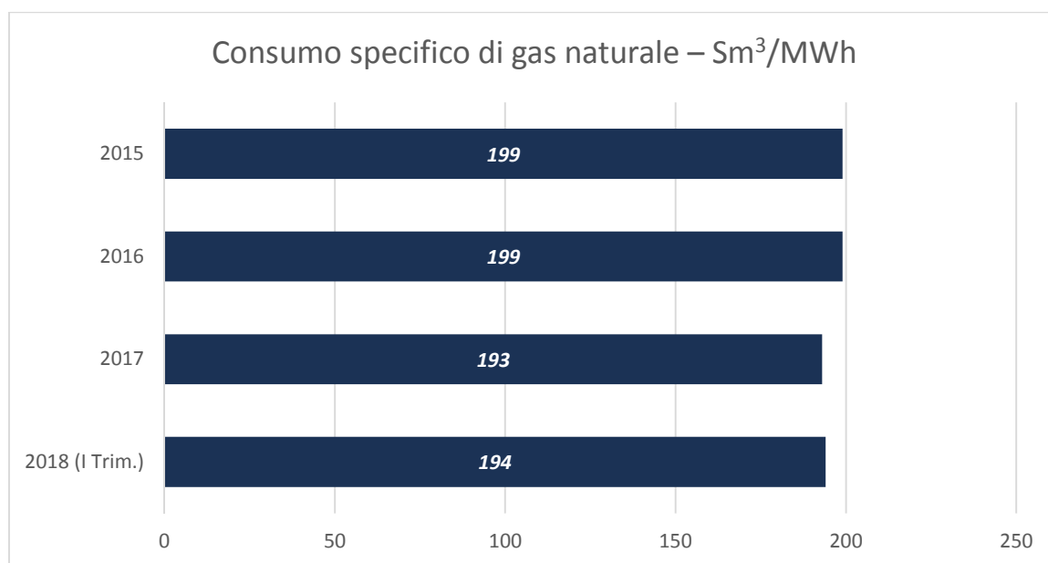
Grafico 6 – Consumo specifico di gas naturale
