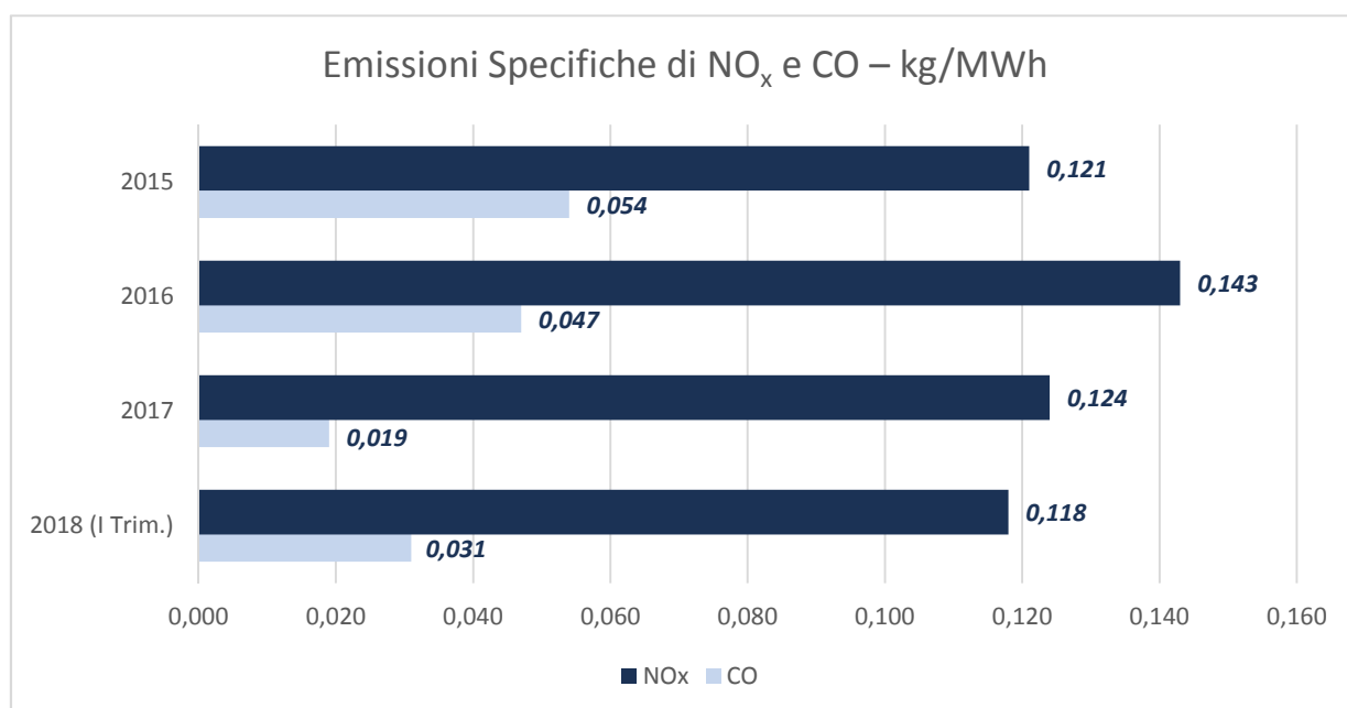
Grafico 5 – Emissioni di NO x e CO
