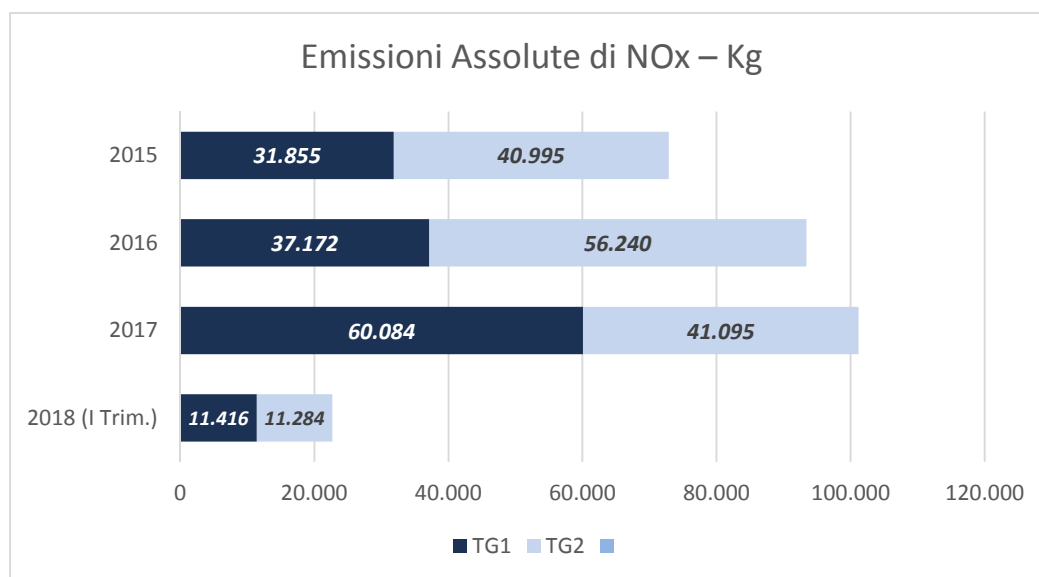
Grafico 1 – Emissioni di \text{NO}_x
