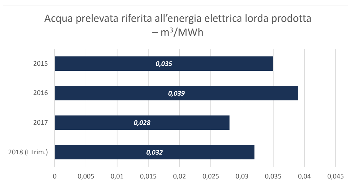
Grafico 11 – Utilizzo di risorsa idrica
